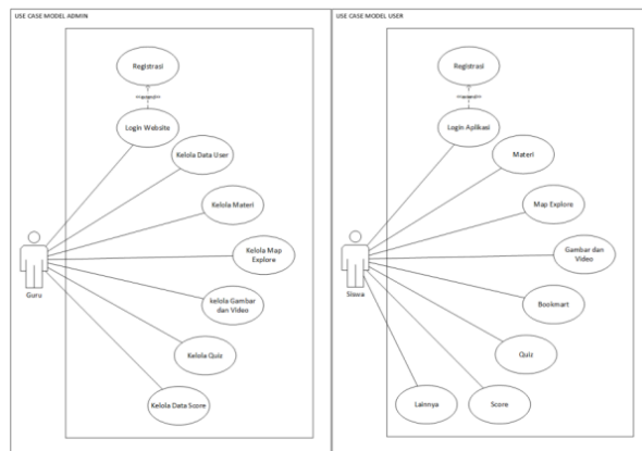
Gambar 1. Usecase Diagram Admin dan User
